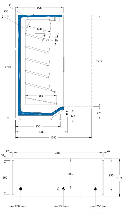
PMM22F3U-nM Multideck Door Meat
