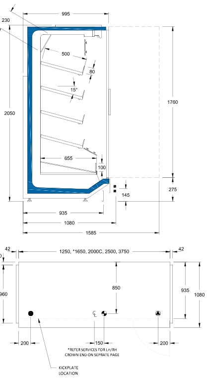
PMM20F3U-nM Multideck Door Meat
