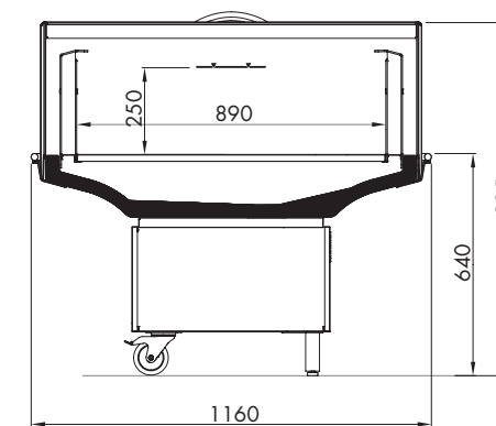
GIANO 90 MAXI GD
