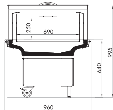
GIANO 70 MAXI GD
